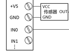
三线制传感器接线
