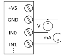
电压电流可同时输入 (仅 3002S、3004S 支持)
