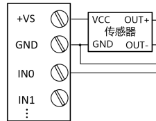
四线制传感器接线
