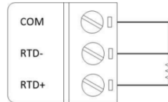
三线制热电阻接线
