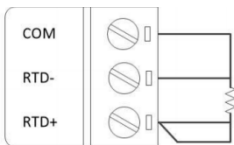
四线制热电阻接线 1
