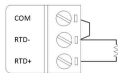
两线制热电阻接线
