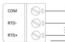
四线制热电阻接线 2
