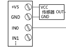
三线制传感器接线
