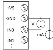
电压电流可同时输入 (仅 3002S、3004S 支持)
