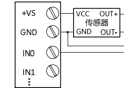
四线制传感器接线
