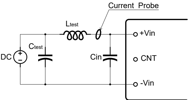
图(10) 输入反射纹波电流测试示意图
