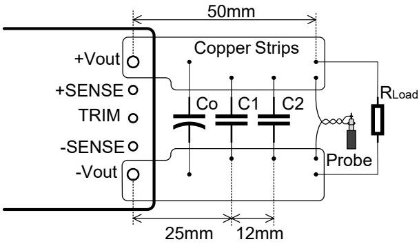
图(11) 输出纹波与噪声测试示意图
