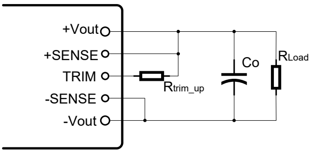
图(12) 输出电压上调节示意图
