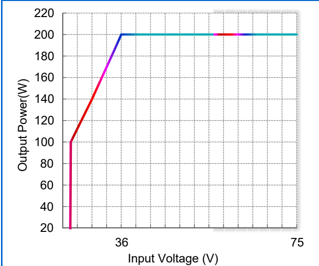
图(7) 全输入电压范围内, 不同输同输入电压下对应的额定输出功率特性曲线.
