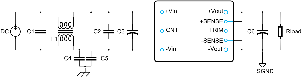
图(9)典型应用电路
