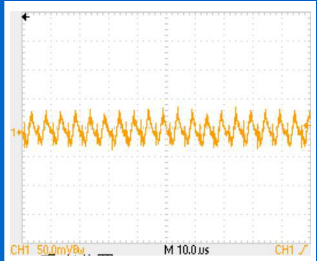
图 (8) 输出端满载时的输出电出电压纹波, 输出端外接 660μF 低ESR电解电容, CH1H1: 50mV/div, 10μs/div.
