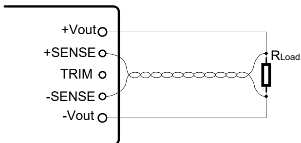
图(14) 输出电压远端补偿电路
