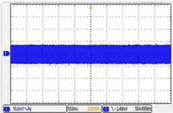
图(11):输出满载时的输出电压纹波 (10ms/div,输出端外接 660 \mu F 固态电容)
