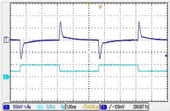
图(9):输出负载阶跃响应波形 (CH1:Vout,CH2:Iout;25%~50%~25%Load,1.0A/ \mu s, 输出端外接 660 \mu F 固态电容)
