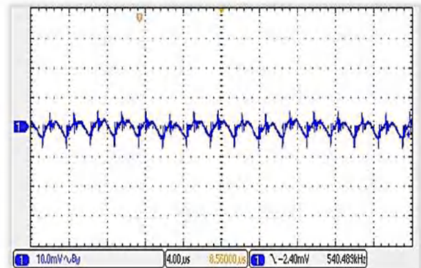
图(12):输出满载时的输出电压纹波 (4 \mu s /div,输出端外接 660 \mu F 固态电容)
