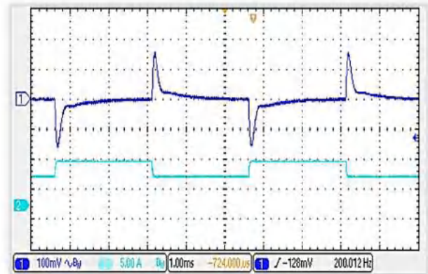
图(10):输出负载阶跃响应波形 (CH1:Vout,CH2:Iout;50%~75%~50%Load,1.0A/ \mu s, 输出端外接 660 \mu F 固态电容)
