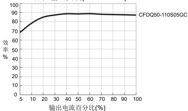
效率/输出负载( V_{in}=110V_{DC} )
