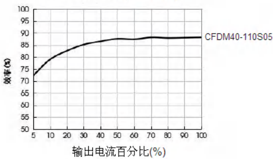
效率/输出负载(Vin=110V)
