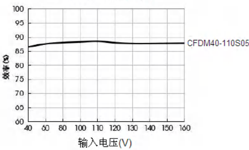
效率/输入电压(满载)
