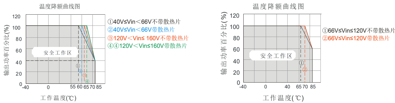
CFDM20-110S05工作温度曲线 图 1
