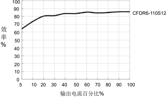
效率/输出负载 (Vin=110VDC)
