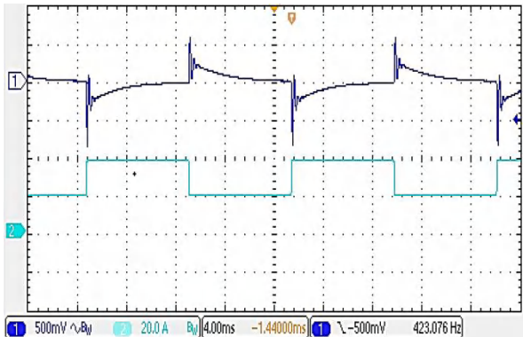
图(9):输出负载阶跃响应波形 (CH1:Vout,CH2:Iout;25%~50%~25%Load,2.5A/ \mu s,输出端外接 1800 \mu F 固态与电解电容)
