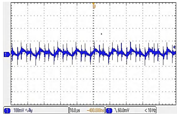
图(12):输出满载时的输出电压高频纹波 (10 \mu s /div 输出端外接 1800 \mu F 低 ESR 电解电容)
