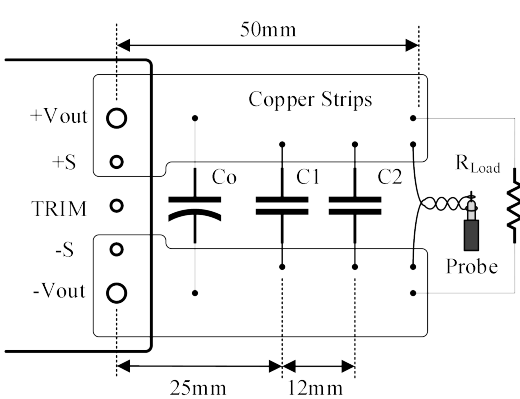
图(15)输出纹波与噪声测试示意图
