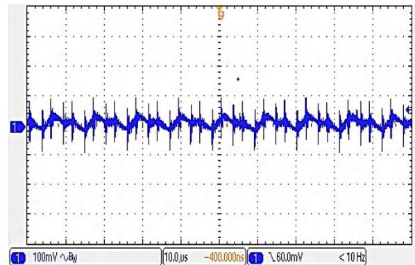
图(12):输出满载时的输出电压高频纹波 (10μs /div 输出端外接 1800μF 低 ESR 电解电容)
