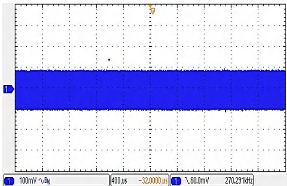
图(11):输出满载时的输出电压低频纹波 (400μs /div,输出端外接 1800μF 低 ESR 电解电容)
