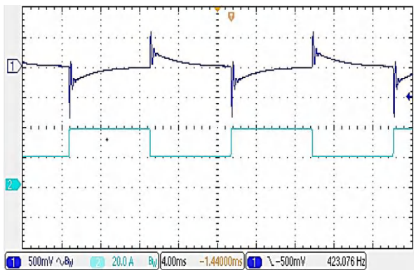
图(9):输出负载阶跃响应波形 (CH1:Vout,CH2:Iout;25%~50%~25%Load,2.5A/μs,输出端外接 1800μF 固态与电解电容)
