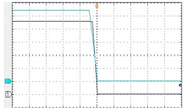
图(6): 输入端断电关机, 输出电压下降波形 (CH1: Vout, CH2: Vin, 输出端满载)
