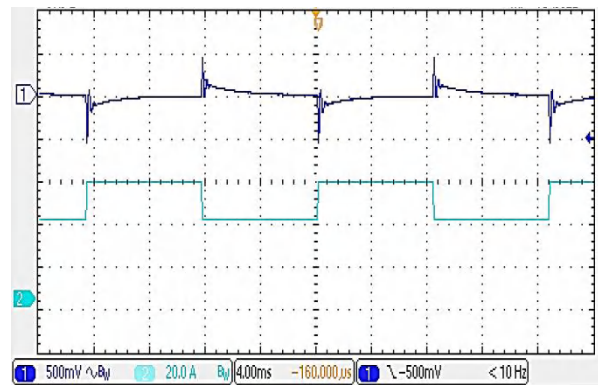
图(10):输出负载阶跃响应波形 (CH1:Vout,CH2:Iout;50%~75%~50%Load, 2.5A/μs,输出端外接 1800μF 固态与电解电容)
