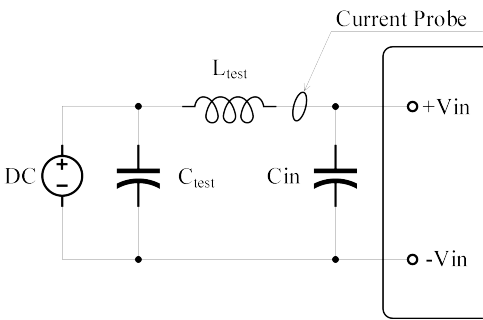
图(14)输入反射纹波电流测试示意图
