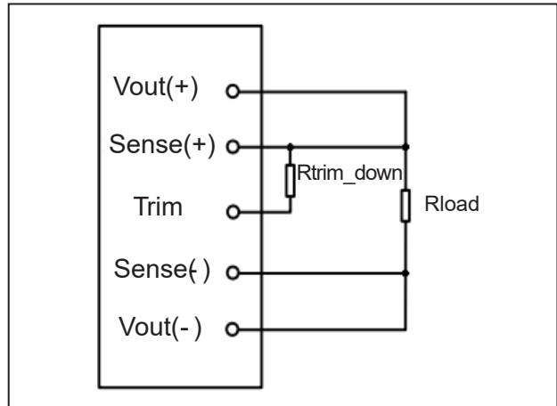
图 H: 输出电压下调示意图
