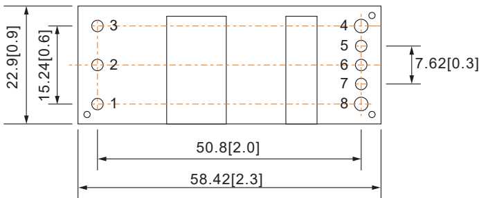
底视图
