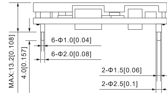
侧视图
