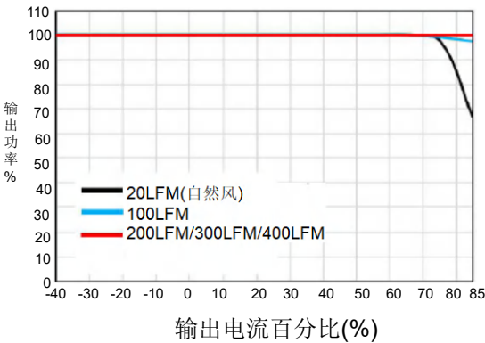
CFDQR75-48S24S温度降额曲线(Vin=24V)
