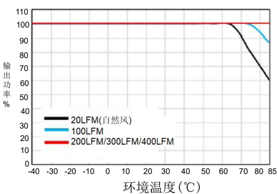
CFDQR75-48S24温度降额曲线(Vin=24V)
