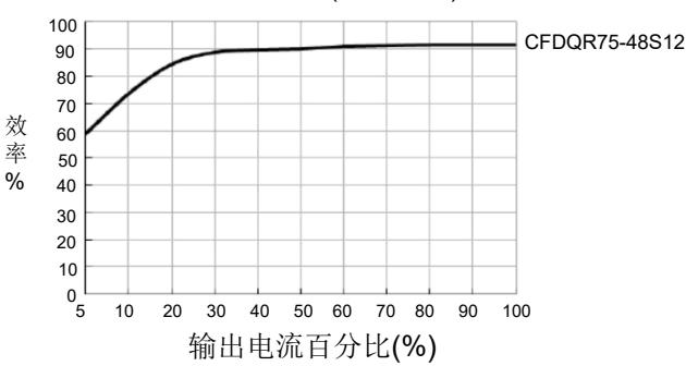
效率/输出负载(Vin=48Vdc)
