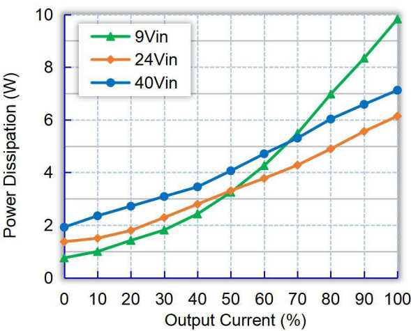
图(2):Tcase=25℃,分别在最小输入电压,额定输入电压,最大输入电压时,不同负载的损耗。
