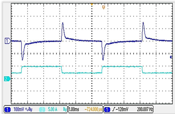
图(9):输出负载阶跃响应波形 (CH1:Vout,CH2:Iout;25%~50%~25%Load,1.0A/μs, 输出端外接 660μF 固态电容)
