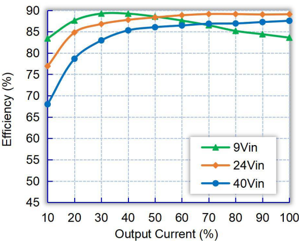
图(1):Tcase=25℃,分别在最小输入电压,额定输入电压,最大输入电压时,不同负载的效率曲线。
