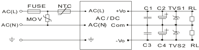
图2:正负双路供地系列典型应用电路
