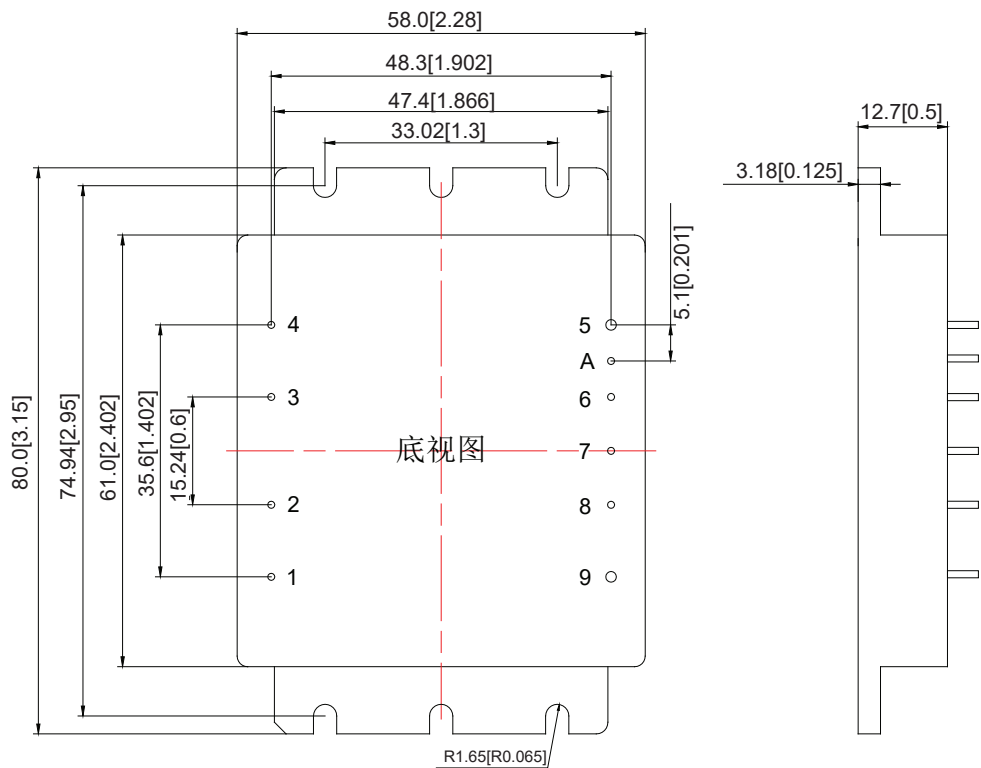
金属外壳带法兰安装孔外观尺寸(单位:mm[英寸])
