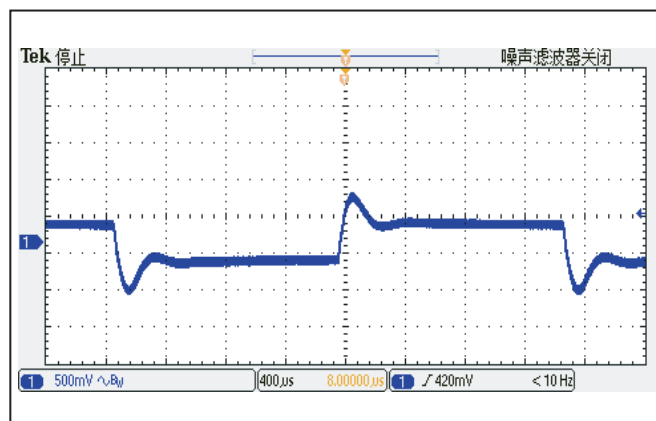
图 4: 负载动态响应, Vin=280V DC , Io:28.6A , Io=50%-75%-50% 2.5A/μs, TC=25°C, CH1: 输出电压
