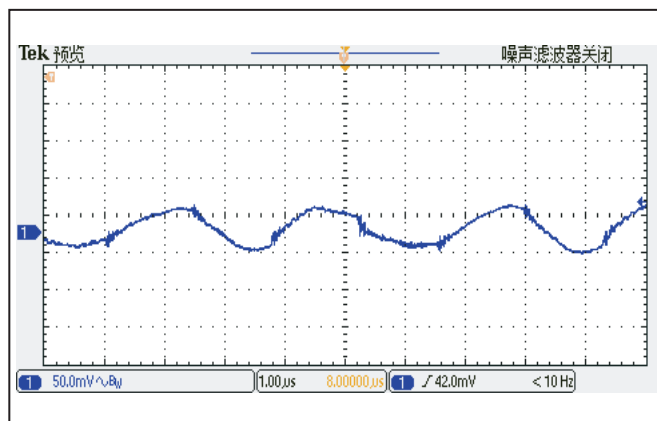
图 3: 输出纹波电压, Vin=280V DC , Io=28.6A, TC=25°C
