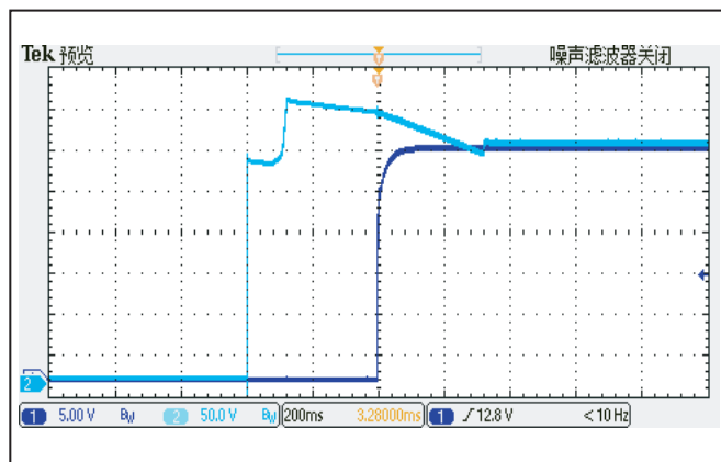
图 5: 启机延时, Vin=280V DC , Io:28.6A TC=25°C CH1: 输出电压, CH2: 输入电压
