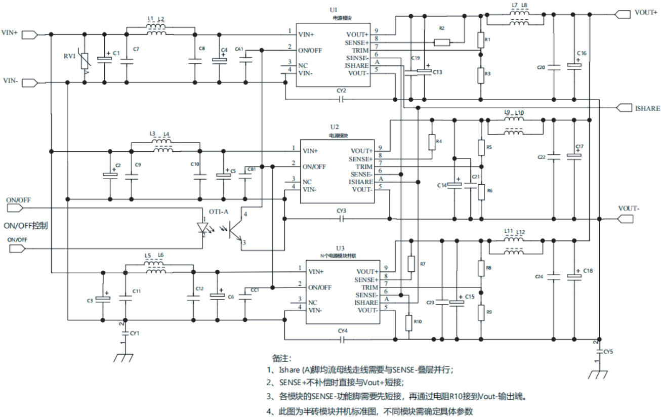
图 B: 典型并联应用电路
