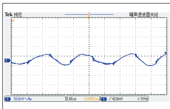
图 3: 输出纹波电压, Vin=280VDC, Io=33.4A, TC=25°C
