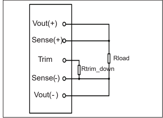
图 I: 输出电压下调示意图
