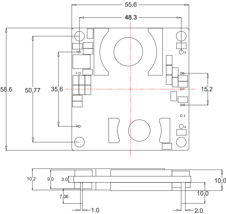
开放式架构外观尺寸(单位:mm)
