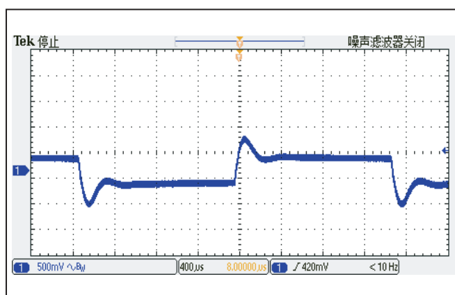
图 4: 负载动态响应, Vin=280VDC, Io=33.4A Io=50%-75%-50% 2.5A/µs, TC=25°C, CH1: 输出电压
