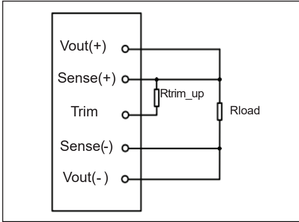
图 H: 输出电压上调示意图
