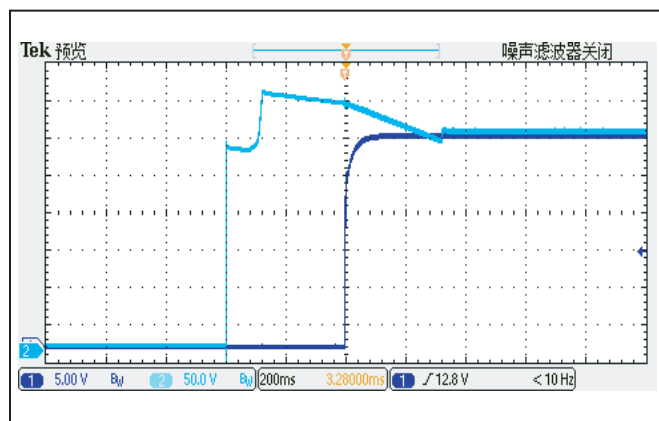
图 5: 启机延时, Vin=280VDC, Io=33.4A TC=25°C CH1: 输出电压, CH2: 输入电压
