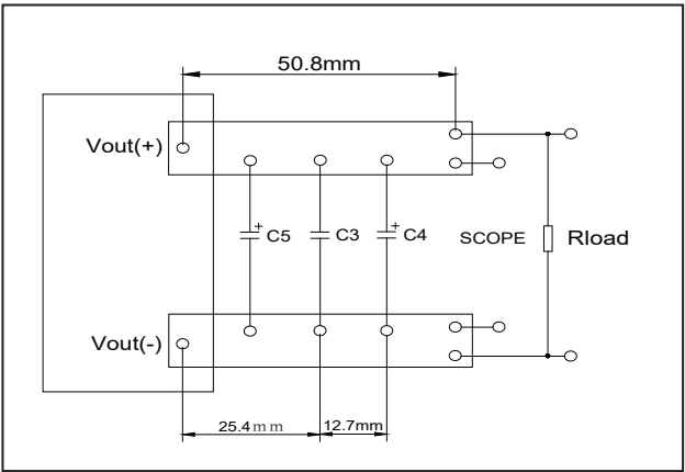
图 G: 输出纹波与噪声测试示意图
