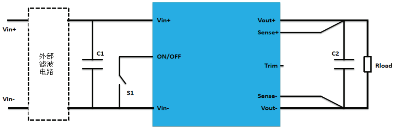
图 A: 典型应用电路
