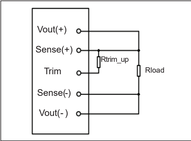
图 H: 输出电压上调示意图
