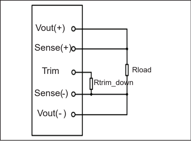
图 I: 输出电压下调示意图
