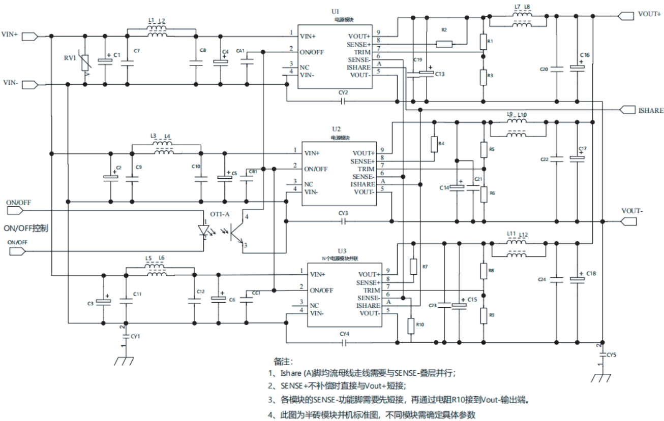
图 B: 典型并联应用电路
