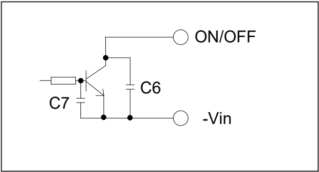
图 D: 晶体管控制方式
