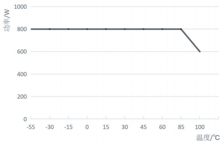
图1：功率-温度降额曲线
