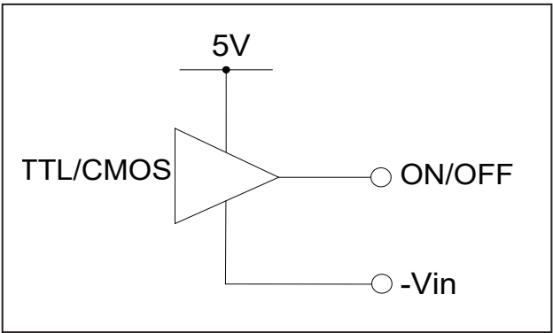
图 F: TTL/CMOS 控制方式
