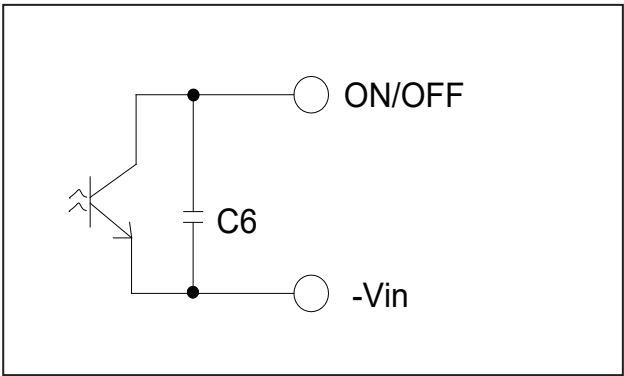
图 E: 隔离控制方式
