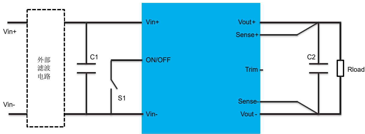
图 A: 典型应用电路
