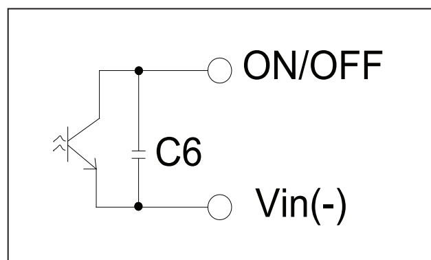
图 D: 隔离控制方式
