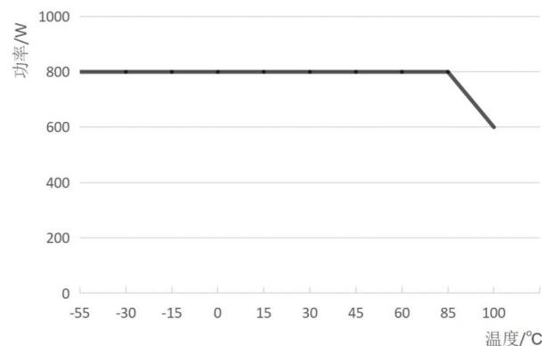
图 1: 功率 - 温度降额曲线
