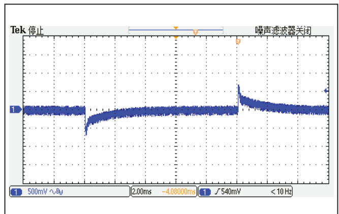
图 4: 负载动态响应, Vin=28V, Io=50%-75%-50%, 2.5A/µS, TC=25°C, CH1: 输出电压
