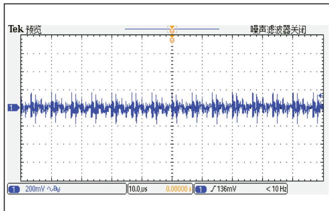
图 3: 输出纹波电压, Vin=28V, Io=66.7A, TC=25°C
