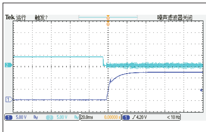
图 5: 启机延时, Vin=28V, TC=25°C CH1: 输出电压, CH2: 输入电压
