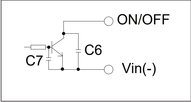
图 D: 晶体管控制方式
