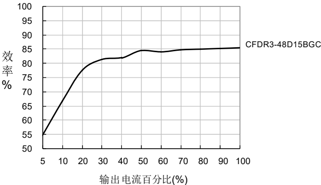
效率/输出负载 (Vin=48V DC )
