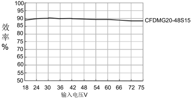
效率/输入电压(满载)
