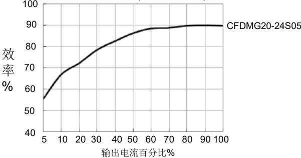
效率/输出负载(Vin=24V DC )
