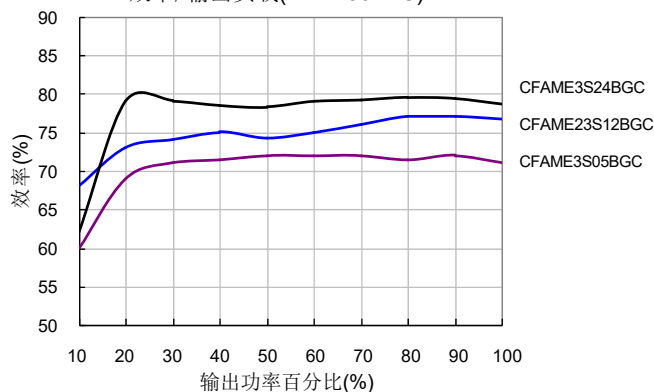
效率/输出负载(Vin=230VAC)
