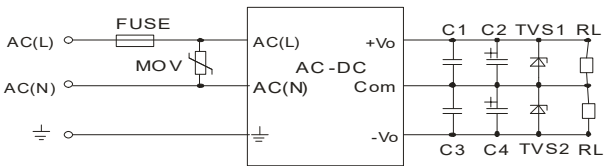
图2: 正负双路典型应用电路
