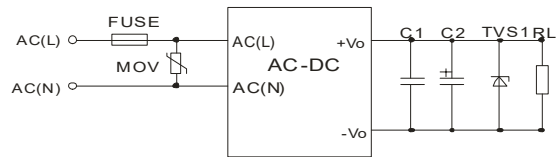
图1: 单路典型应用电路
