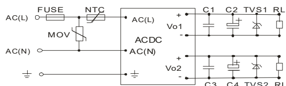
图3:双隔离双路系列典型应用电路
