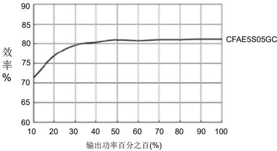
效率/输出负载(Vin=230VAC)
