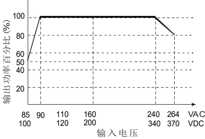
输入电压降额曲线图
