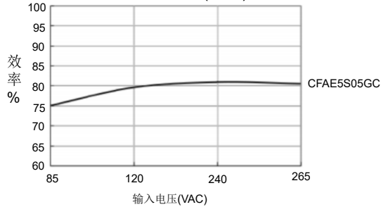
效率/输入电压(满载)
