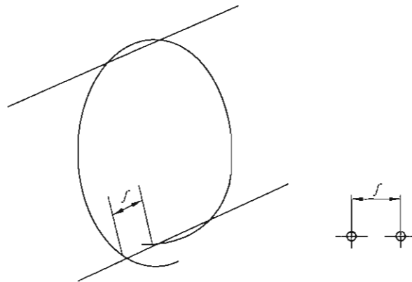
图 1 钢丝的圈形
